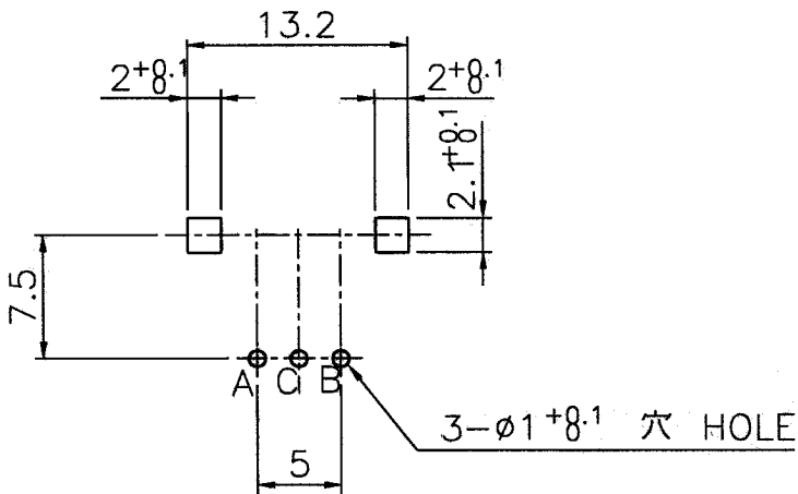
기판두께 t = 1.6mm P.C.B. HOLE LAY OUT
