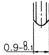
단자 선단 상세도 (8 : 1) TERMINAL DETAIL (8 : 1)
